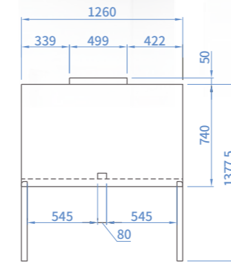
SFT45-2G SFT45-4G
