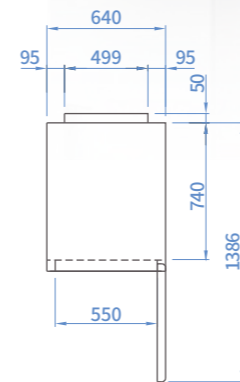
SFT25-1G SFT25-2G
